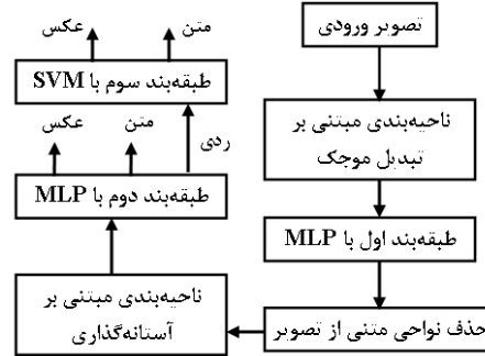
شکل (۲): روند نمای طبقه بندی سلسله مراتبی مبتنی بر ناحیه بندی [۱] Fig. (2): The general process of classifying the sequences based on regioning [1]
