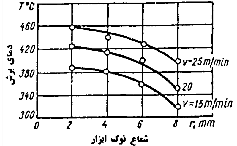
اثر شعاع ابزار بر روی درجه حرارت برش
