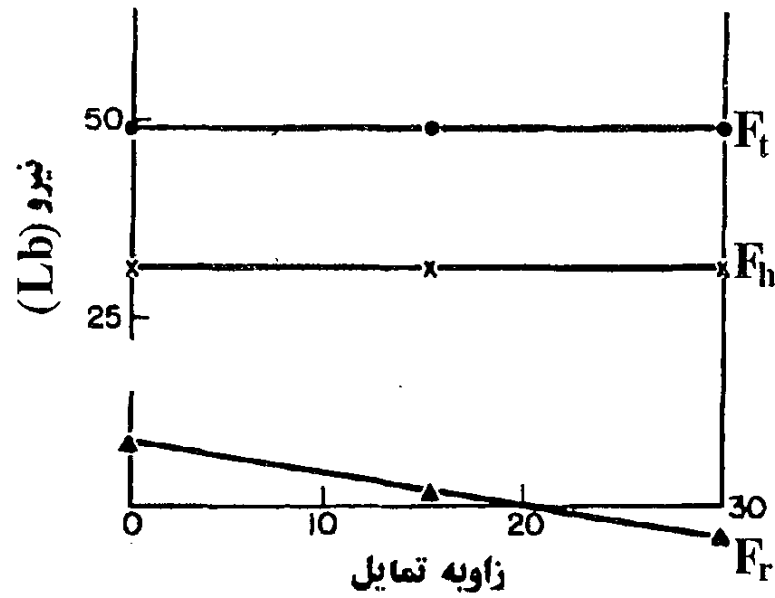
اثر زاویه تمایل بر نیروهای برش
