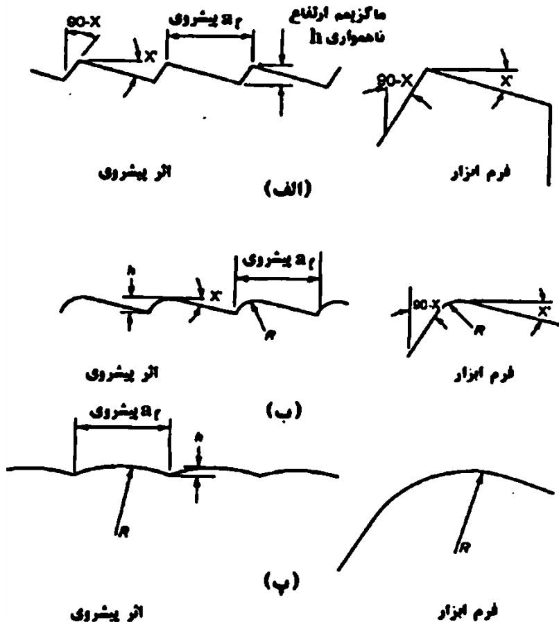
اثر شکل هندسی ابزار بر زبری سطح
