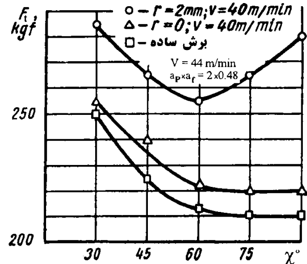
اثر زاویه تنظیم اصلی بر نیروی اصلی تراش
