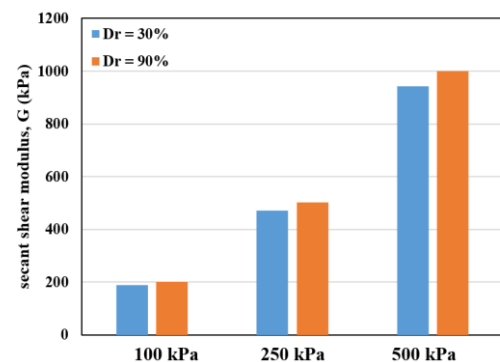
شکل ۲۹- تغییرات مدول برشی سکانتی ماسه کربناته
