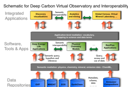
شکل ۵- شماتیک ساختار شبکه مجازی اکتشاف کربن در اعماق زمین[4]
