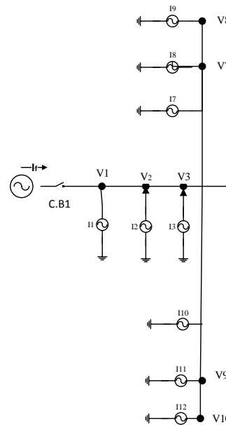
شکل (۵). شمای تک خطی شبکه شبیه سازی شده با نفوذ بالای منابع PV.
