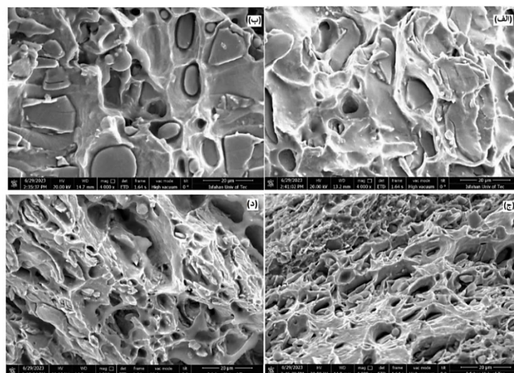
شکل 9- تصاویر SEM از سطح شکست نمونه‌ها بعد از انجام فرایند FSP بدون ذرات تقویت کننده الف - و کامپوزیت Cu-Ag-SiC با ذرات تقویت کننده SiC همراه با ب - 0/02 گرم و ج - 0/04 گرم ذرات میکرونی و د - ذرات نانومتری
