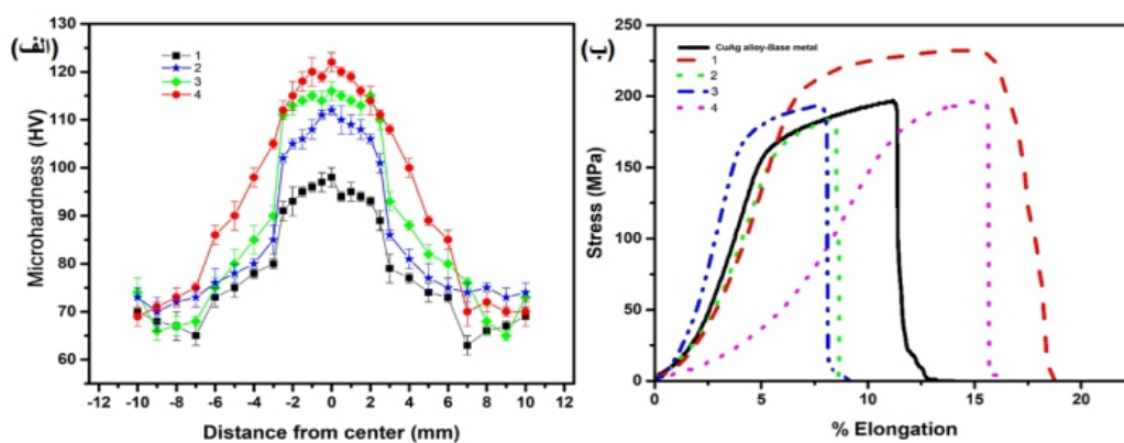
شکل 8-الف - نمودار ریزسختی سنجی و یکرز نمونه FSP شده بدون ذرات تقویت کننده (نمونه 1)، کامپوزیت
