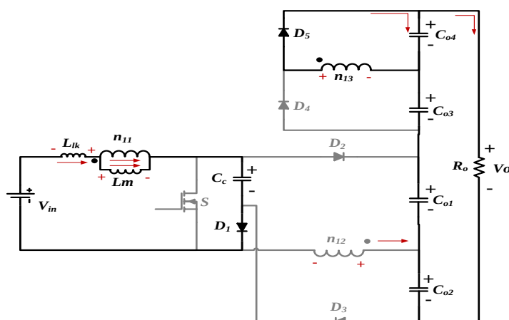
شکل (۵): مبدل پیشنهادی در وضعیت دوم عملکرد
