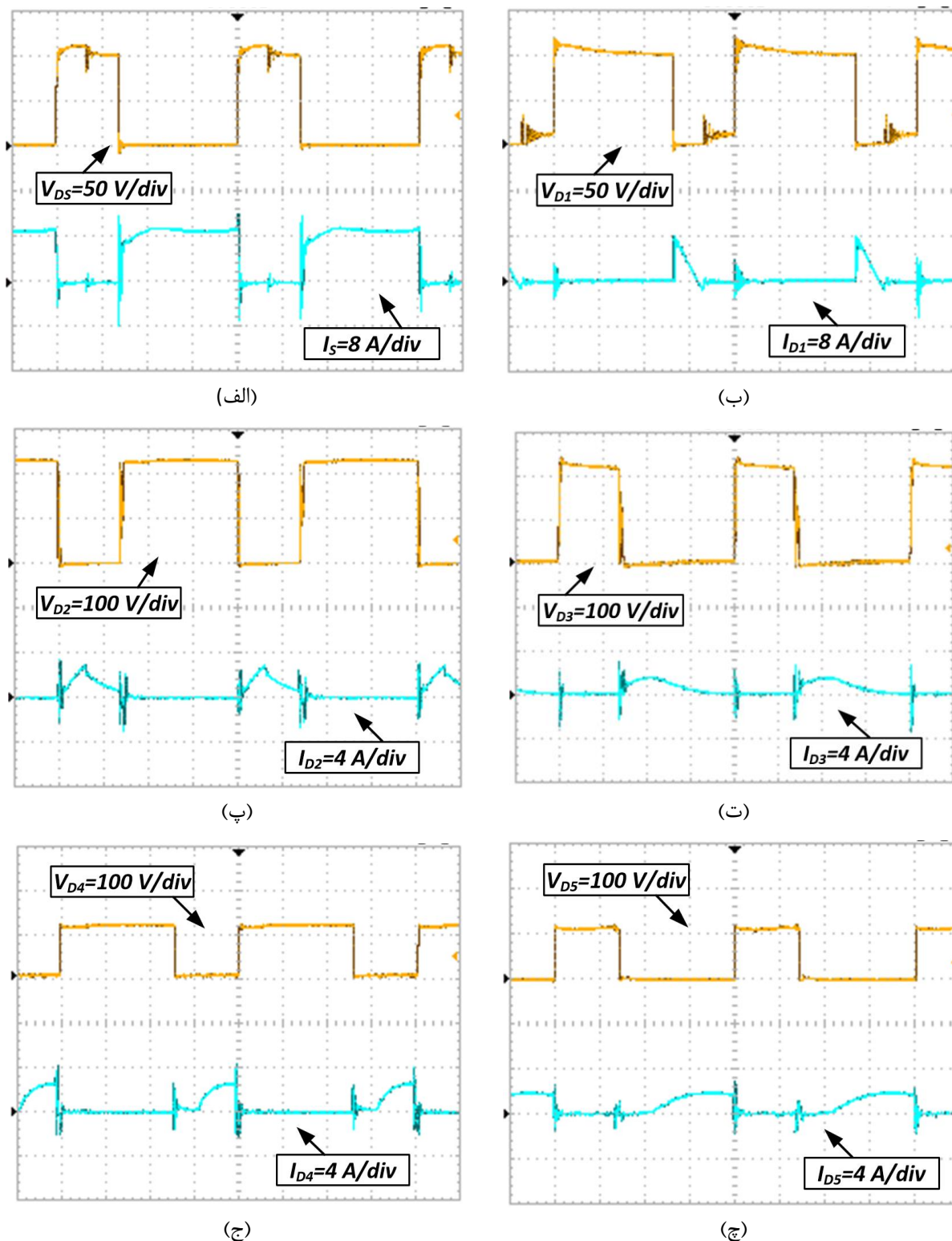
شکل (۱۲) شکل موج‌های عملی مبدل پیشنهادی
